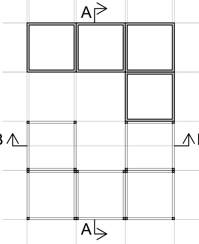
PLANTA NIVEL 0
