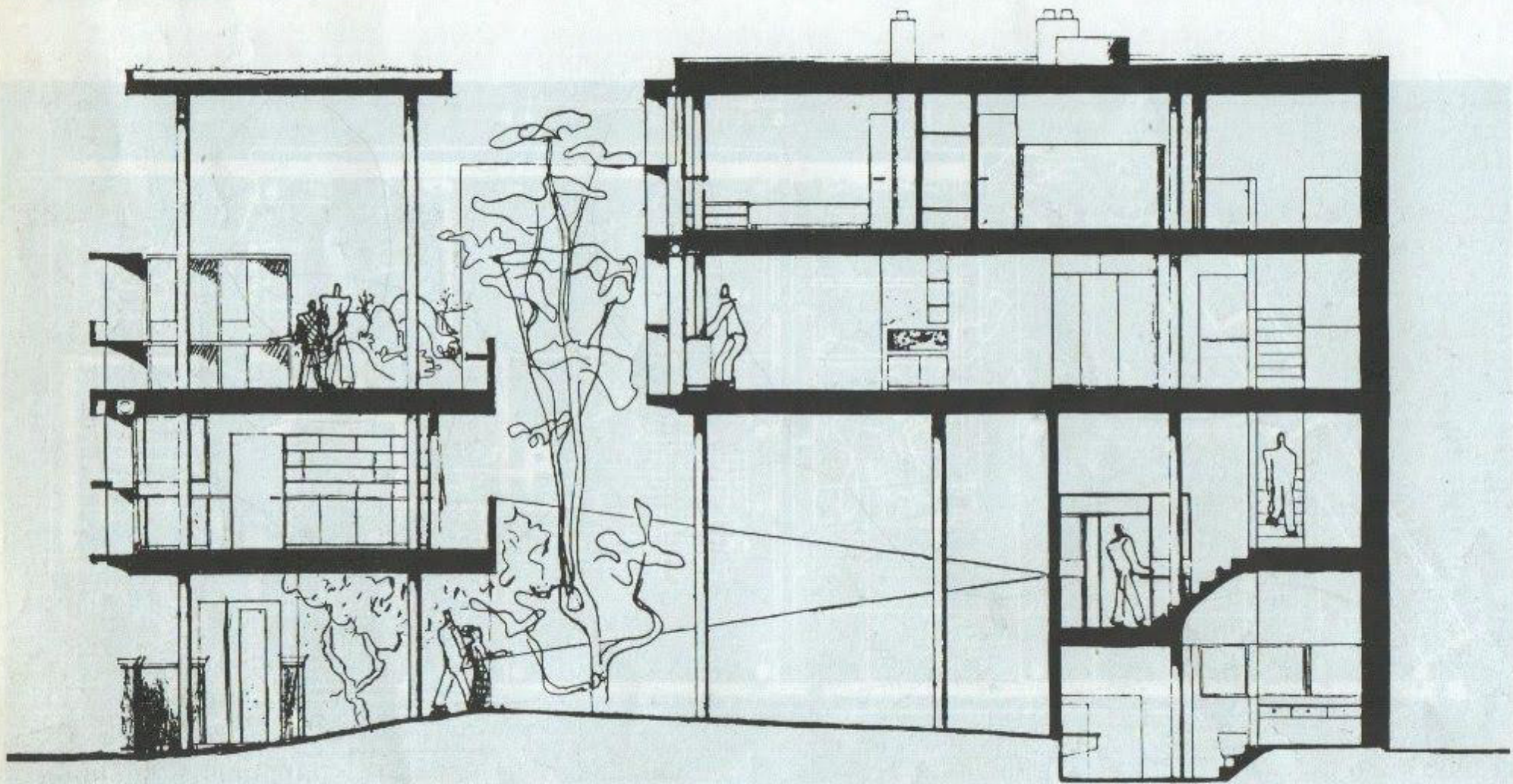
Coupe longitudinale côté rampe
